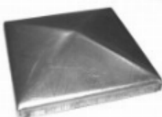
Заглушка, арт. 15.059 150x150x1мм Вес: 0.25 кг Цена: 96 руб.
