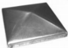
Заглушка, арт. 15.056 80x80x1мм Вес: 0.076 кг Цена: 18,50 руб.
