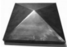
Заглушка на столб 80x80, арт. 15.056.02 80x80x1мм Вес: 0.079 кг Цена: 21 руб.
