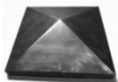
Заглушка на столб 120x120, арт. 15.058.02 120x120x1мм Вес: 0.142 кг Цена: 48 руб.
